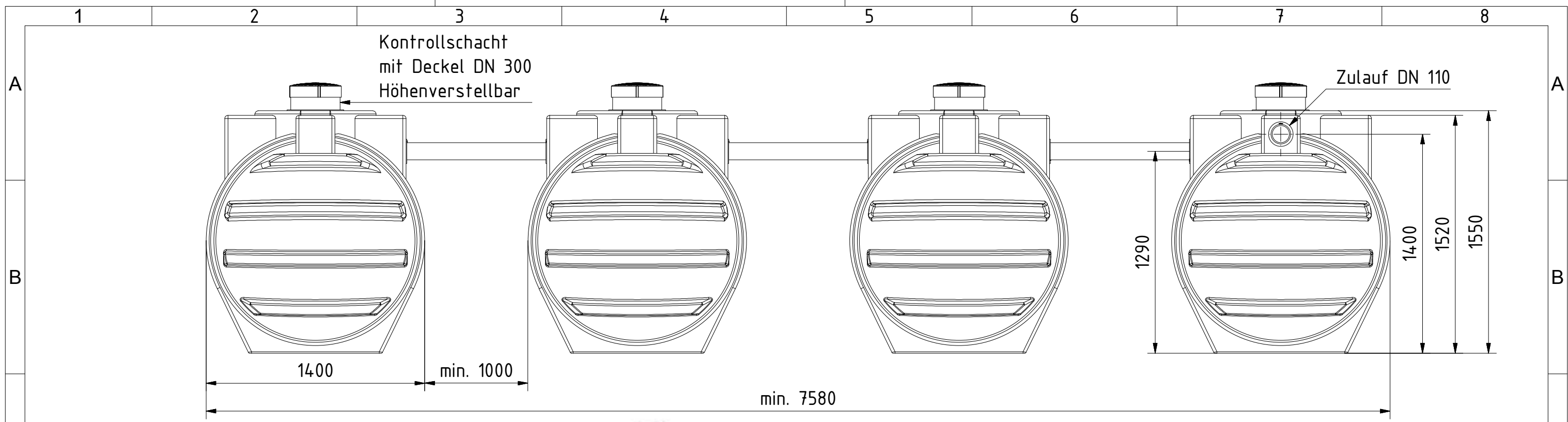
Frontansicht
